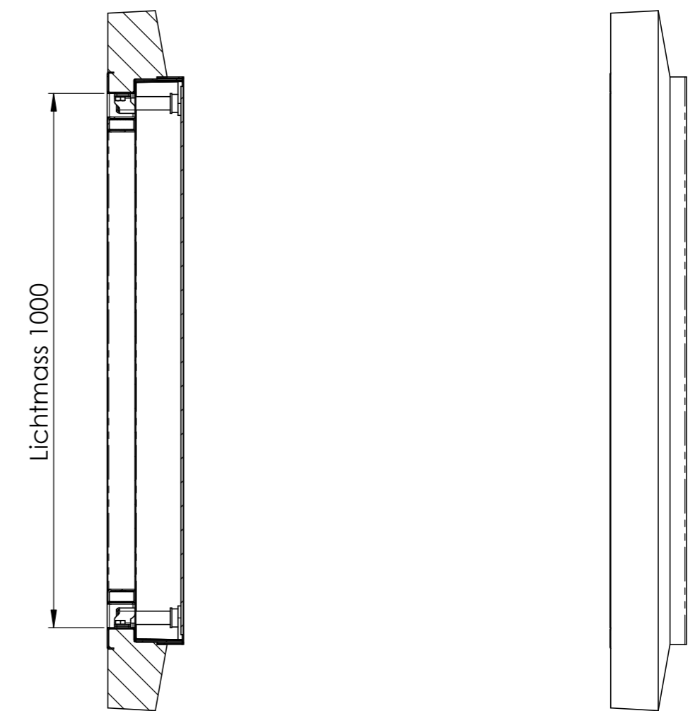
SCHNITT B-B
